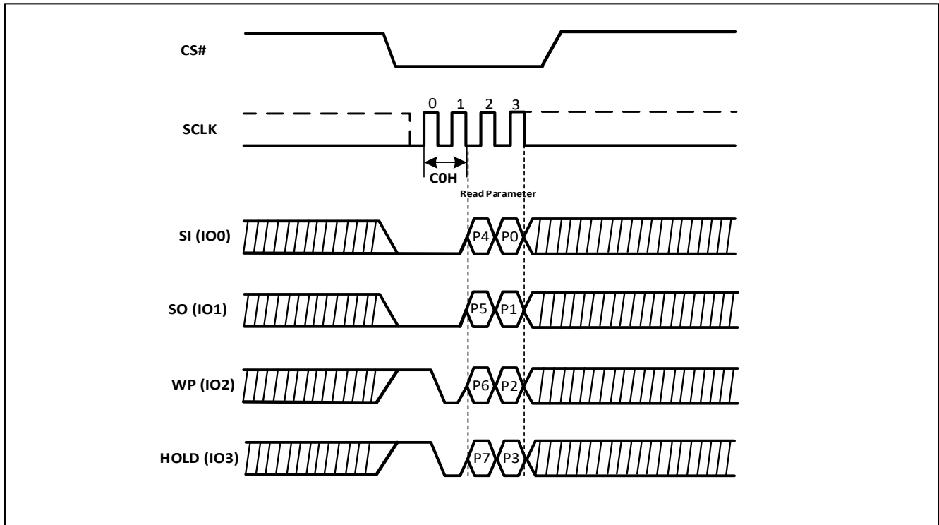
Figure-31. Set Read Parameters (QPI)
